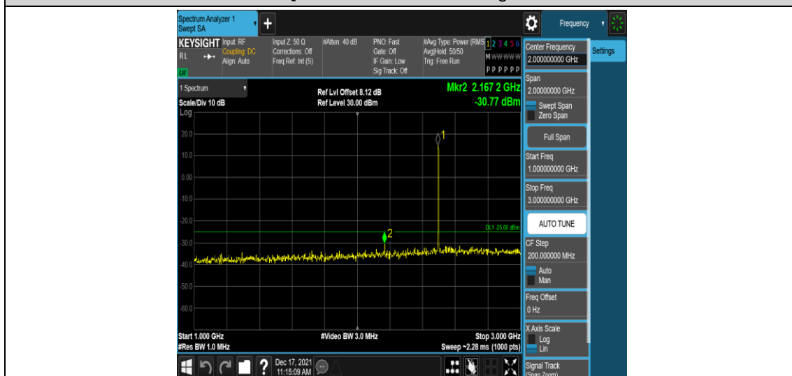
Band41-5MHz-QPSK-39675-1RB#0-Range4:1000~3000MHz
