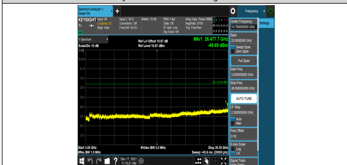
Band41-5MHz-QPSK-39675-1RB#0-Range5:3000~26500MHz
