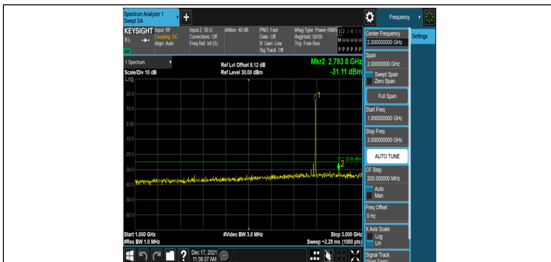
Band41-10MHz-QPSK-40620-1RB#0-Range4:1000~3000MHz
