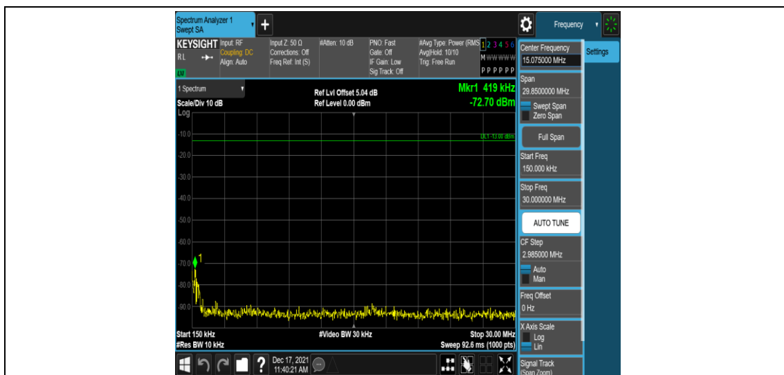
Band41-10MHz-QPSK-41540-1RB#0-Range2:0.15~30MHz
