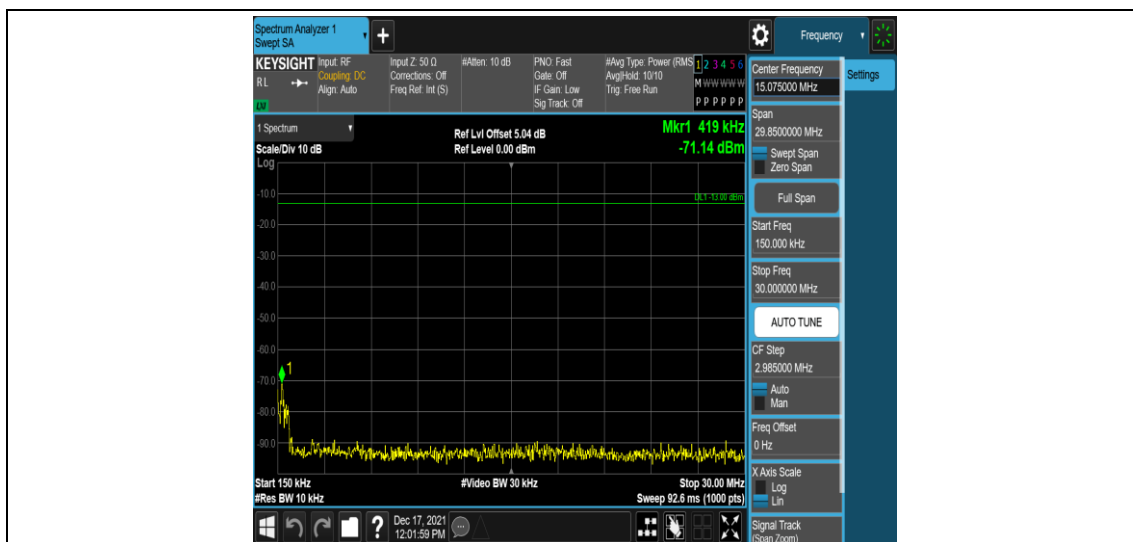
Band41-15MHz-QPSK-41515-1RB#0-Range2:0.15~30MHz
