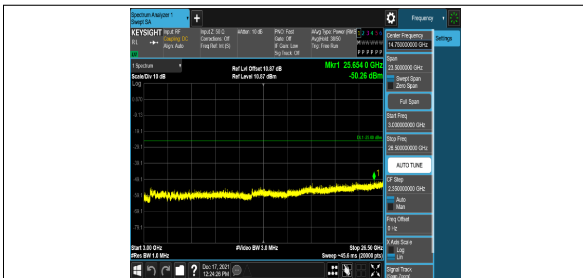
Band41-20MHz-QPSK-41490-1RB#0-Range5:3000~26500MHz
