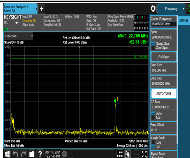
Band41-20MHz-QPSK-40620-1RB#0-Range2:0.15~30MHz
