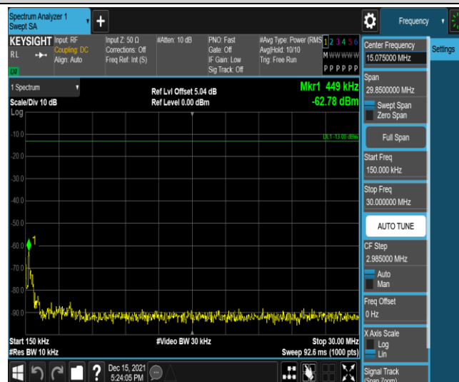
Band5-1.4MHz-QPSK-20525-1RB#0-Range2:0.15~30MHz
