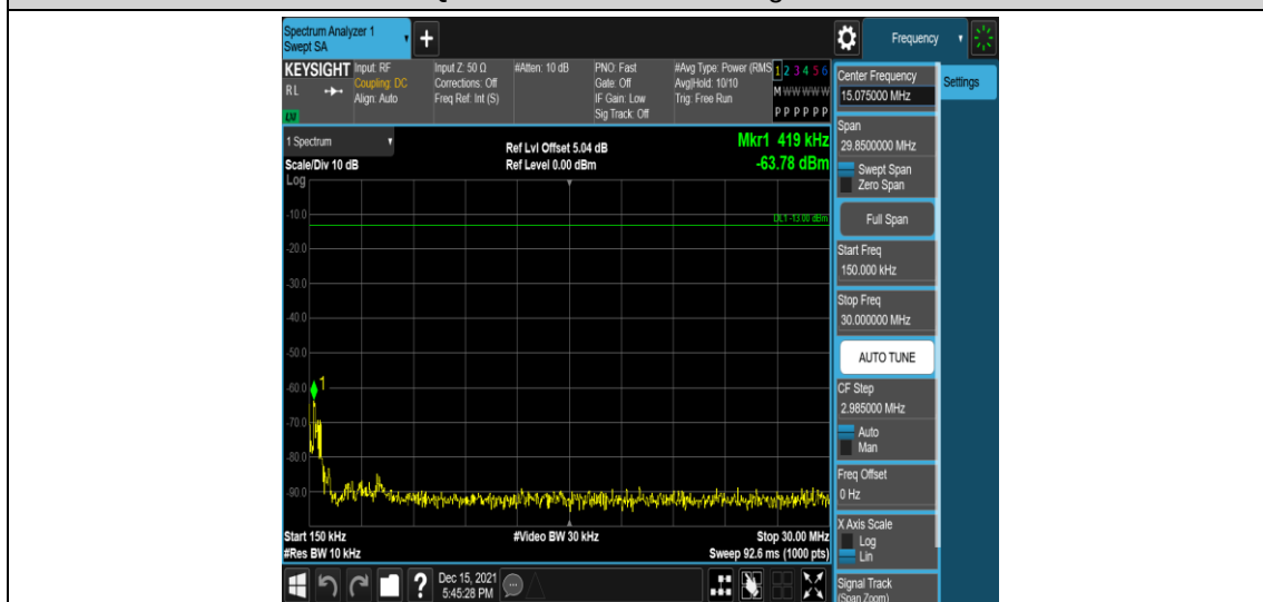
Band5-3MHz-QPSK-20635-1RB#0-Range2:0.15~30MHz
