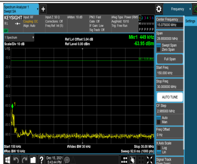
Band5-3MHz-QPSK-20525-1RB#0-Range2:0.15~30MHz
