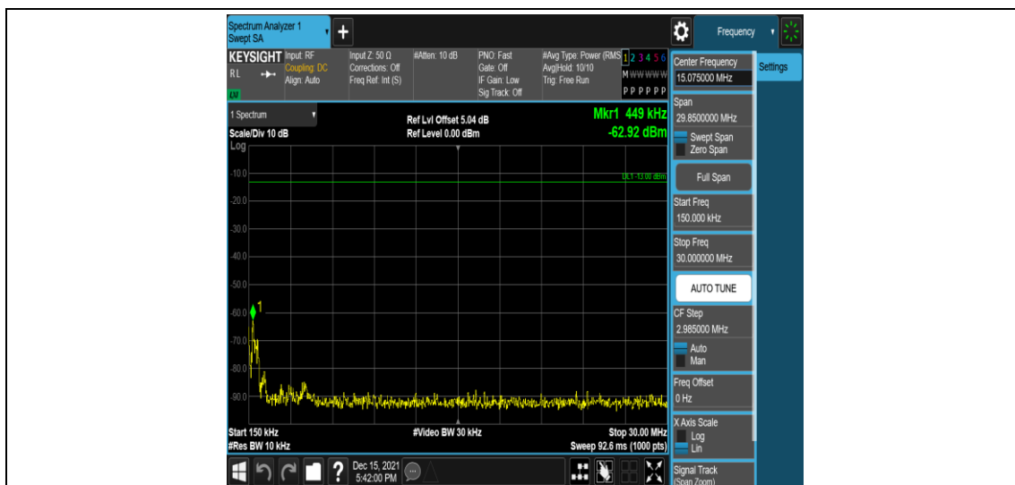
Band5-3MHz-QPSK-20415-1RB#0-Range2:0.15~30MHz
