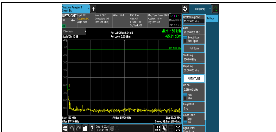
Band66-3MHz-QPSK-131987-1RB#0-Range2:0.15~30MHz
