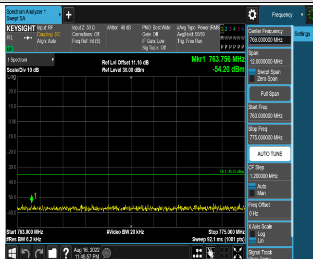
Band13-5MHz-QPSK-23255-1RB#0-Range5:763~775MHz
