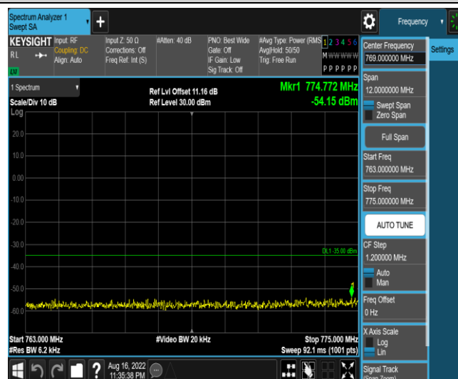
Band13-5MHz-QPSK-23205-1RB#0-Range5:763~775MHz
