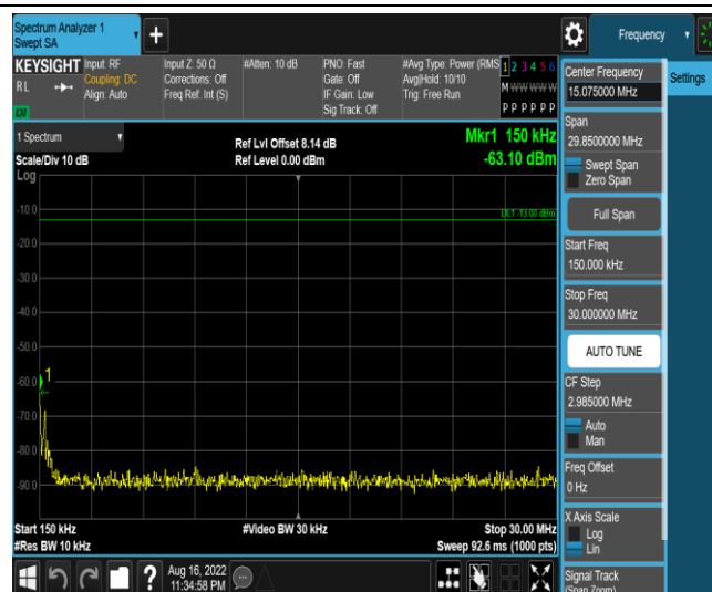
Band13-5MHz-QPSK-23205-1RB#0-Range2:0.15~30MHz
