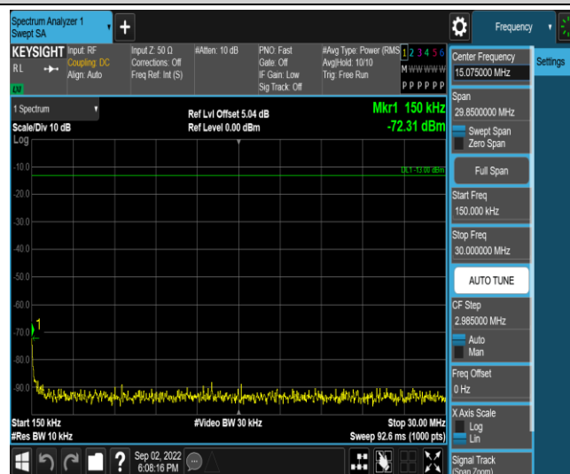
Band2-3MHz-16QAM-19185-1RB#0-Range2:0.15~30MHz
