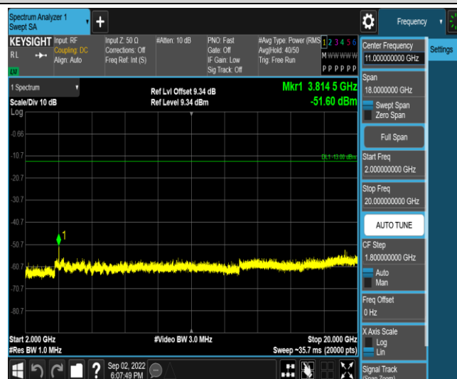
Band2-3MHz-QPSK-19185-1RB#0-Range5:2000~20000MHz
