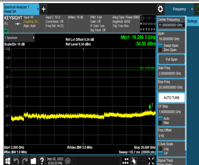
Band2-3MHz-QPSK-18615-1RB#0-Range5:2000~20000MHz
