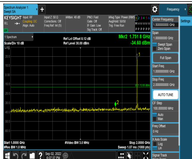
Band2-3MHz-QPSK-19185-1RB#0-Range4:1000~2000MHz
