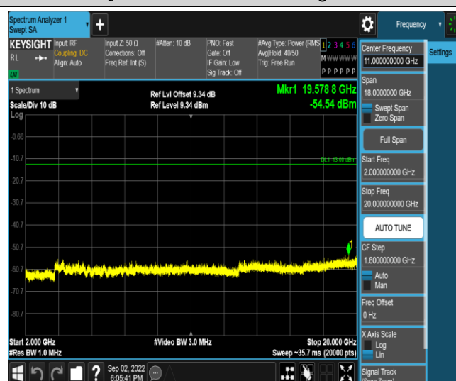
Band2-3MHz-QPSK-18900-1RB#0-Range5:2000~20000MHz
