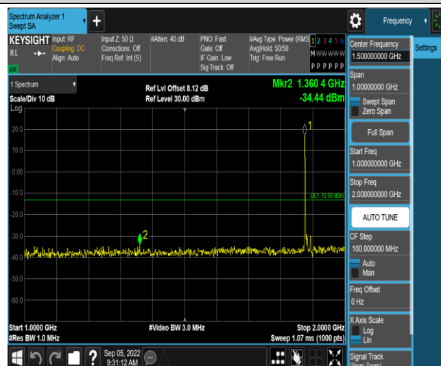
Band2-10MHz-QPSK-18900-1RB#0-Range4:1000~2000MHz
