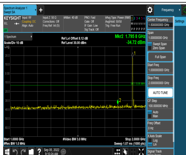
Band2-5MHz-16QAM-19175-1RB#0-Range4:1000~2000MHz
