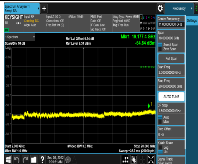
Band2-5MHz-QPSK-19175-1RB#0-Range5:2000~20000MHz
