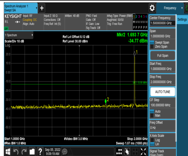
Band2-5MHz-QPSK-19175-1RB#0-Range4:1000~2000MHz
