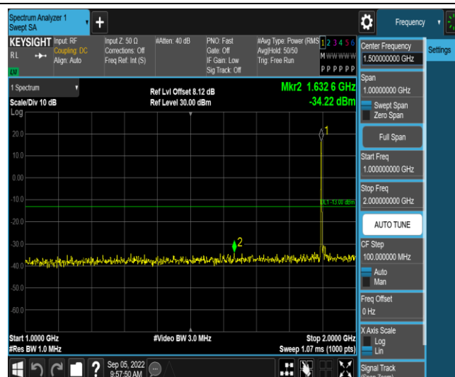
Band2-15MHz-QPSK-19125-1RB#0-Range4:1000~2000MHz
