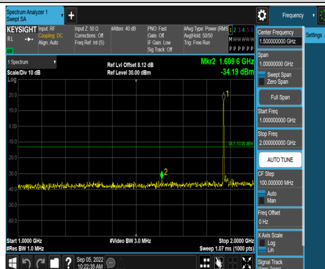
Band2-20MHz-16QAM-18900-1RB#0-Range4:1000~2000MHz
