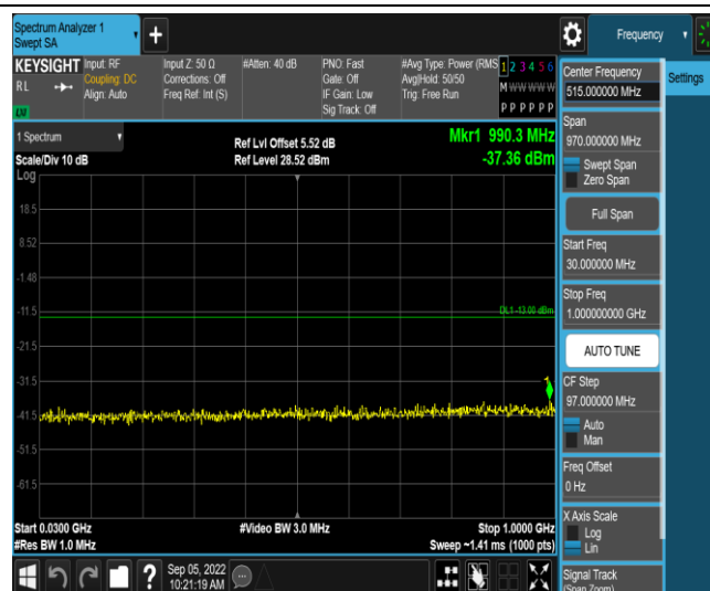
Band2-20MHz-QPSK-18900-1RB#0-Range3:30~1000MHz
