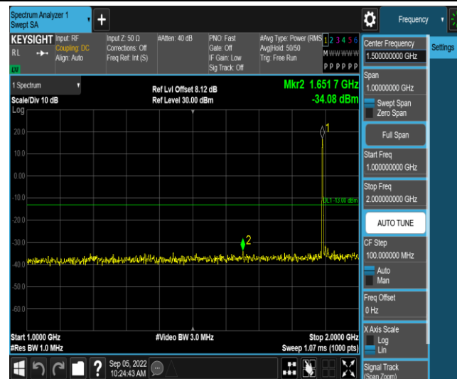
Band2-20MHz-16QAM-19100-1RB#0-Range4:1000~2000MHz
