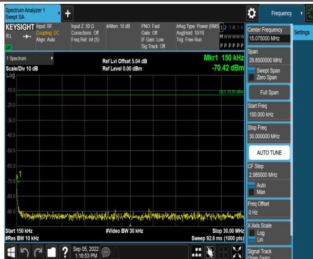
Band25-3MHz-QPSK-26675-1RB#0-Range2:0.15~30MHz
