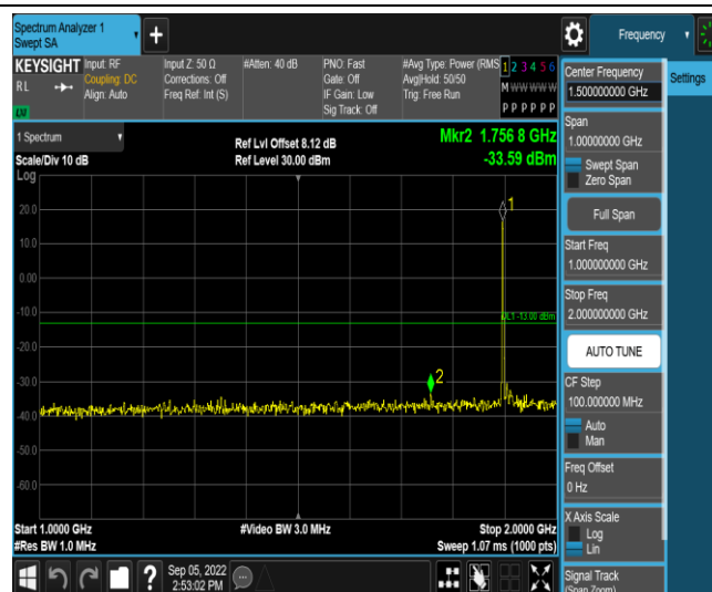
Band25-20MHz-QPSK-26590-1RB#0-Range4:1000~2000MHz
