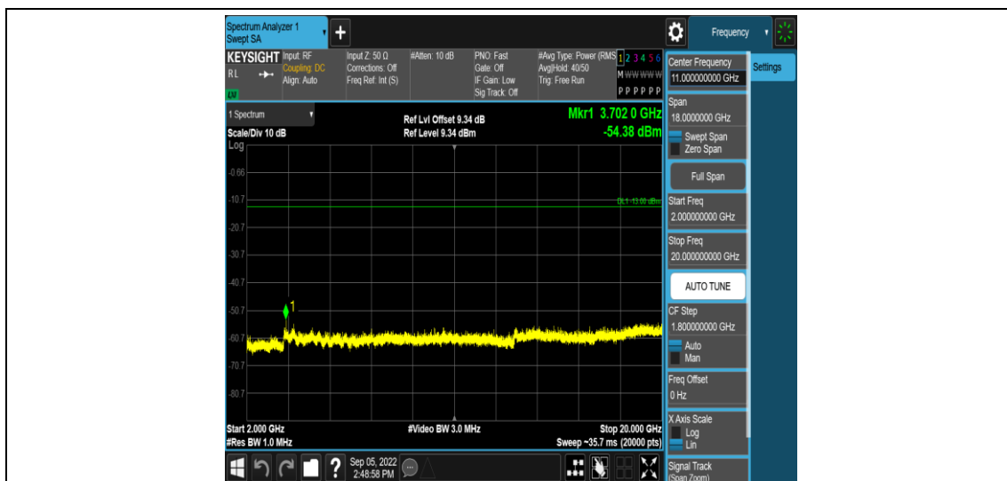
Band25-20MHz-QPSK-26140-1RB#0-Range5:2000~20000MHz
