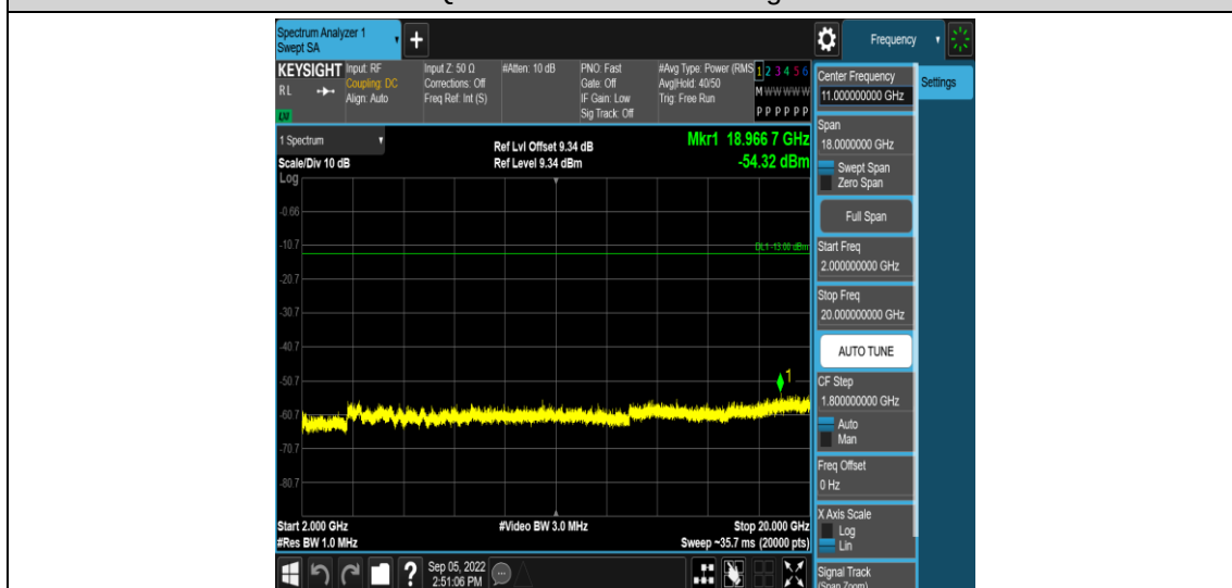
Band25-20MHz-QPSK-26365-1RB#0-Range5:2000~20000MHz
