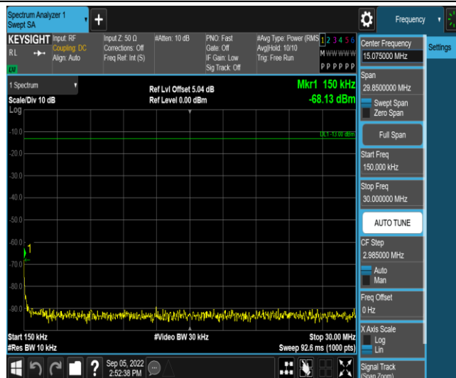
Band25-20MHz-QPSK-26590-1RB#0-Range2:0.15~30MHz
