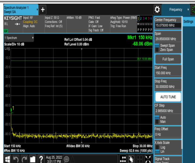
Band26-5MHz-QPSK-26815-1RB#0-Range2:0.15~30MHz
