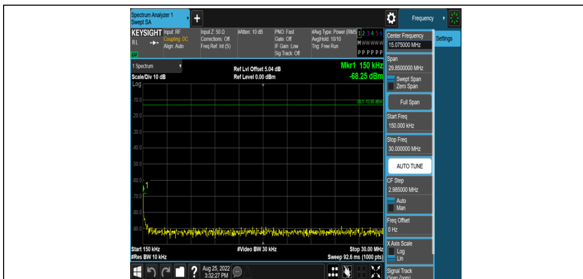
Band26-3MHz-QPSK-26915-1RB#0-Range2:0.15~30MHz
