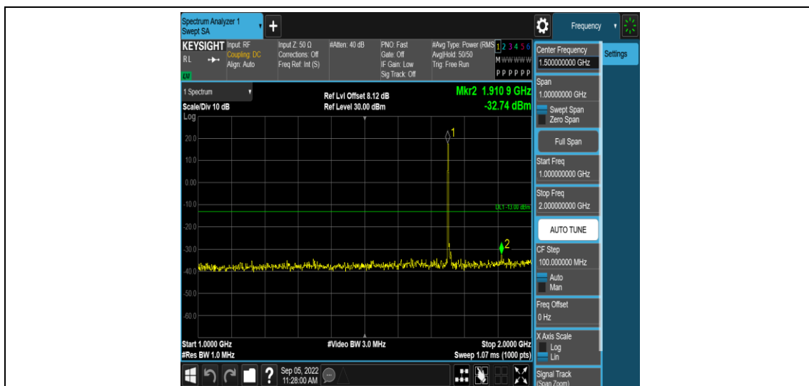
Band4-5MHz-QPSK-20375-1RB#0-Range4:1000~2000MHz
