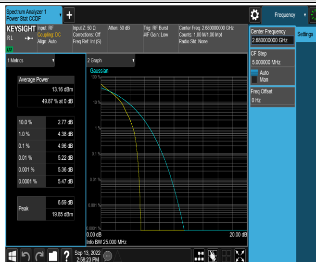
Band41-20MHz-QPSK-41490-1RB#0
