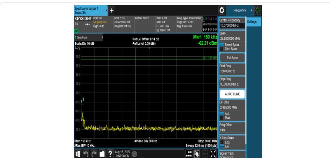
Band5-5MHz-QPSK-20425-1RB#0-Range2:0.15~30MHz
