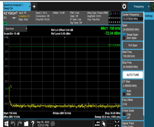
Band66-20MHz-QPSK-132322-1RB#0-Range2:0.15~30MHz
