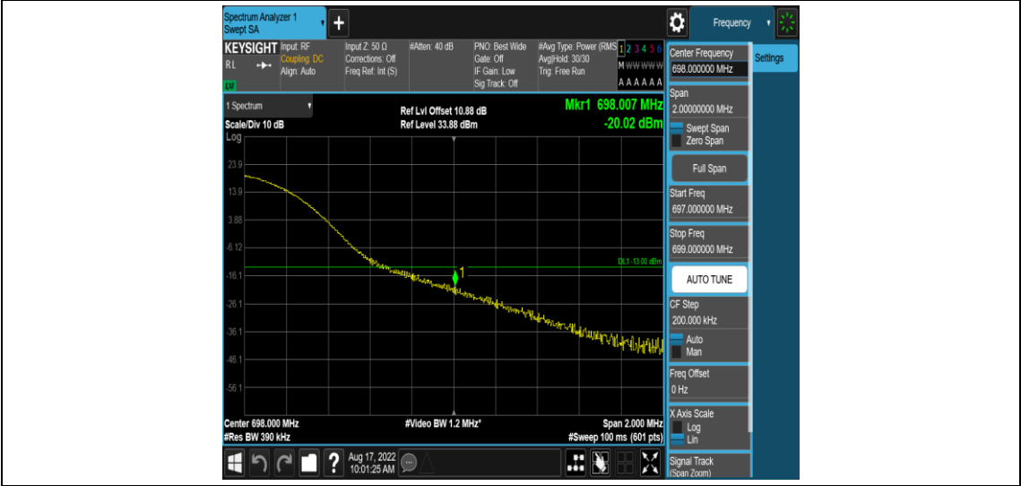
Band71-20MHz-16QAM-133372-1RB#99
