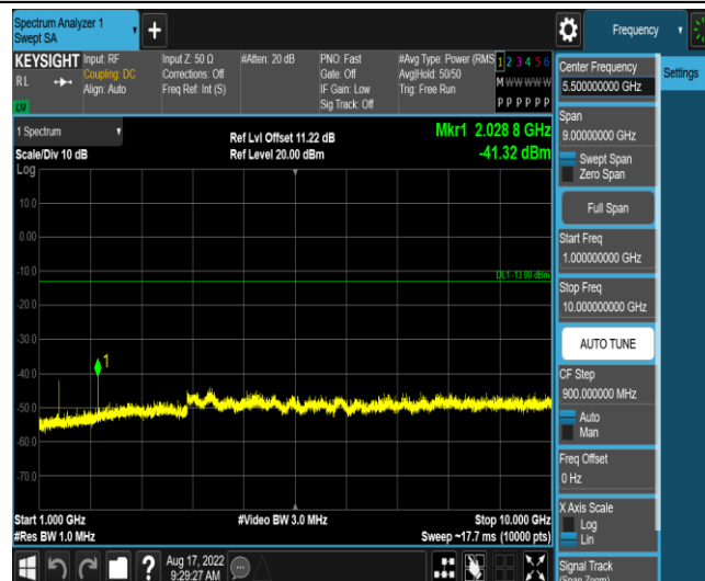
Band71-10MHz-QPSK-133297-1RB#0-Range4:1000~10000MHz
