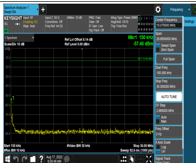
Band71-10MHz-QPSK-133422-1RB#0-Range2:0.15~30MHz
