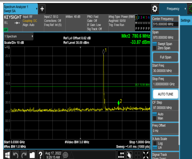
Band71-10MHz-QPSK-133297-1RB#0-Range3:30~1000MHz
