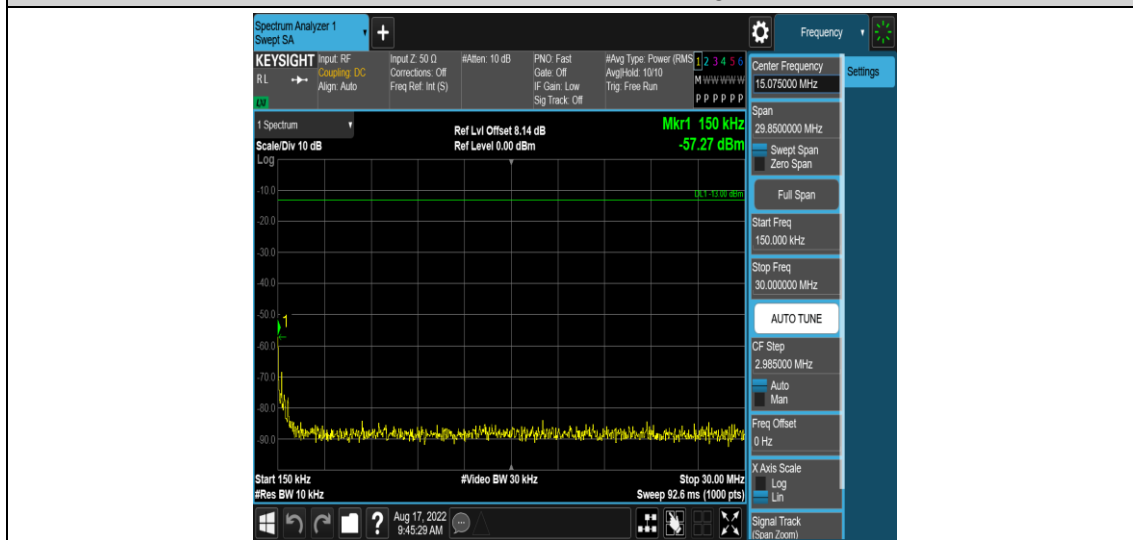
Band71-15MHz-QPSK-133197-1RB#0-Range2:0.15~30MHz
