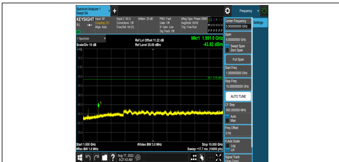
Band71-10MHz-QPSK-133172-1RB#0-Range4:1000~10000MHz
