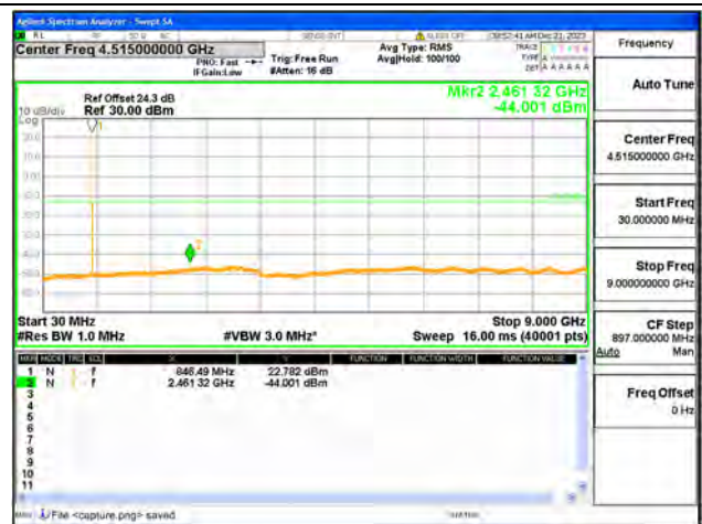
B5 / 3MHz / High CH / QPSK
