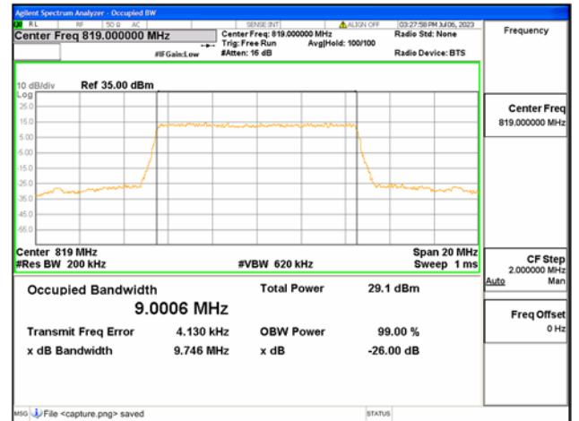
Band26 Part90 / 10MHz / QPSK/ Low CH
