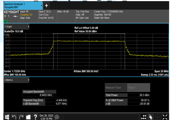
B4 10M 64QAM 50@0 CH 20175
