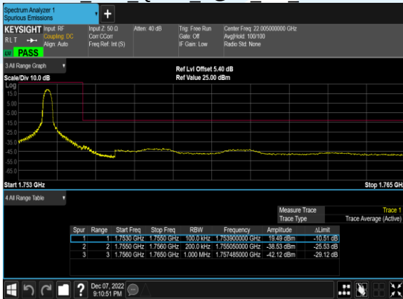
B4 20M 16QAM 1@99 CH 20300
