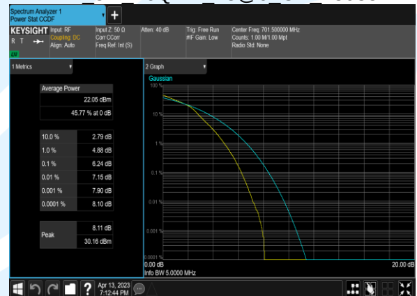
B12_5M 16QAM 25@0 CH 23095
