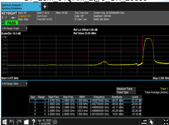
B7 20M 64QAM 1@0 CH 20850
