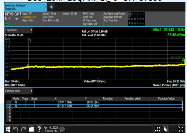
B38 20M 16QAM 1@0 CH 37850
