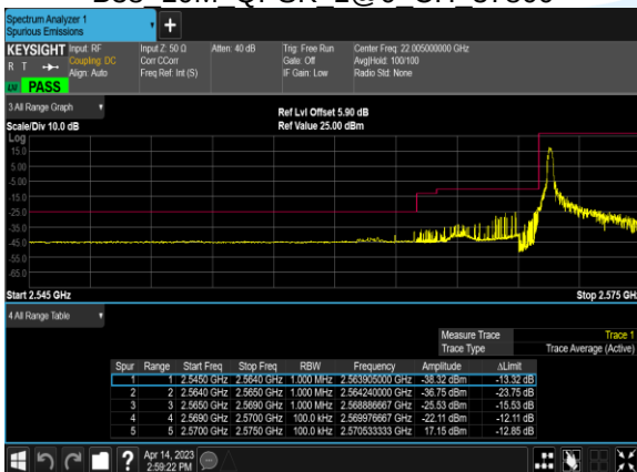
B38 10M QPSK 1@0 CH 37800
