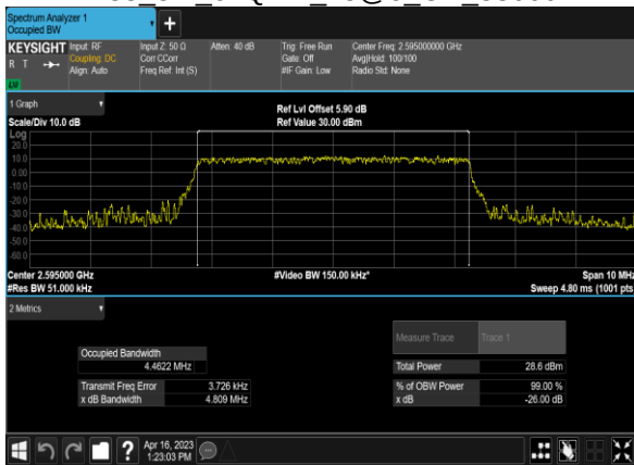
B38 5M 64QAM 25@0 CH 38000
