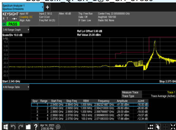
B38 20M QPSK 1@0 CH 37850
