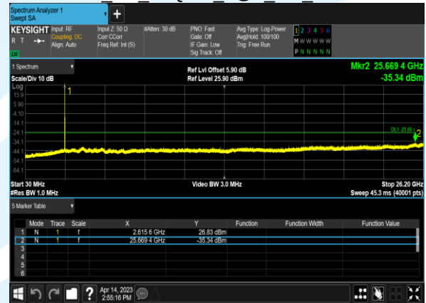
B38 20M 64QAM 1@0 CH 38000
