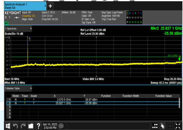
B38 5M 16QAM 1@0 CH 38000
