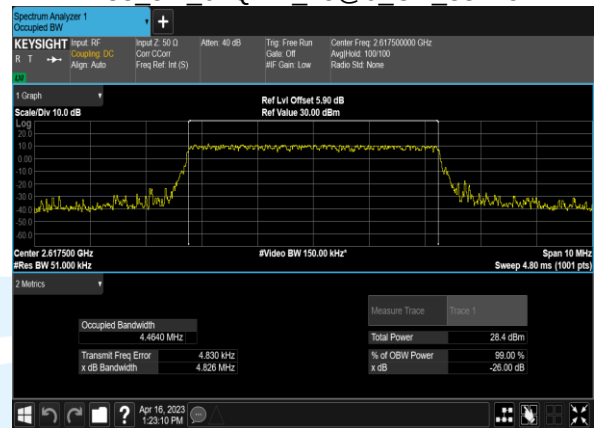
B38 5M 64QAM 25@0 CH 38225
