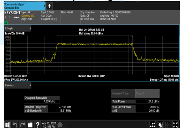
B38 20M 64QAM 100@0 CH 38000
