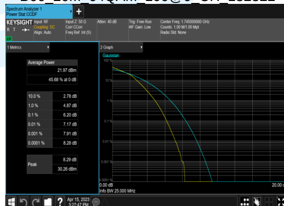
B66 20M 64QAM 100@0 CH 132322
