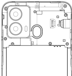
Fente pour la carte SIM
