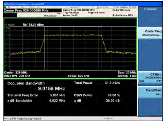
Band5 / 10MHz / QPSK/ Low CH
