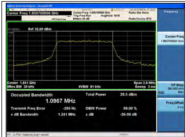
Band2 / 1.4MHz / QPSK/ Low CH
