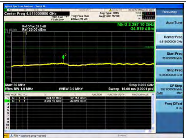
Band5 / 1.4MHz / Low CH / 16QAM
