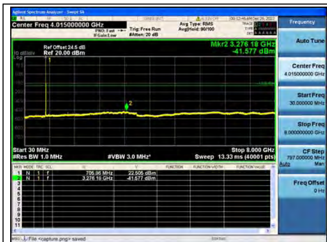
Band17 / 10MHz / Mid CH / QPSK
