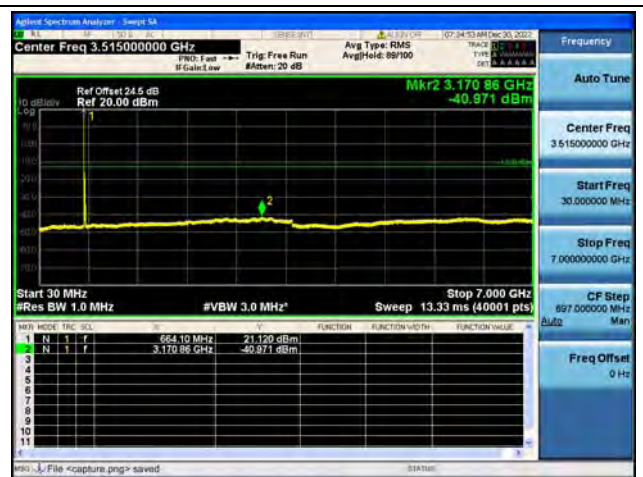
Band71 / 15MHz / Low CH / 16QAM
