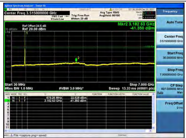
Band71 / 20MHz / High CH / 64QAM
