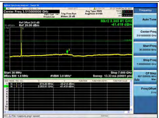
Band71 / 20MHz / Mid CH / 16QAM
