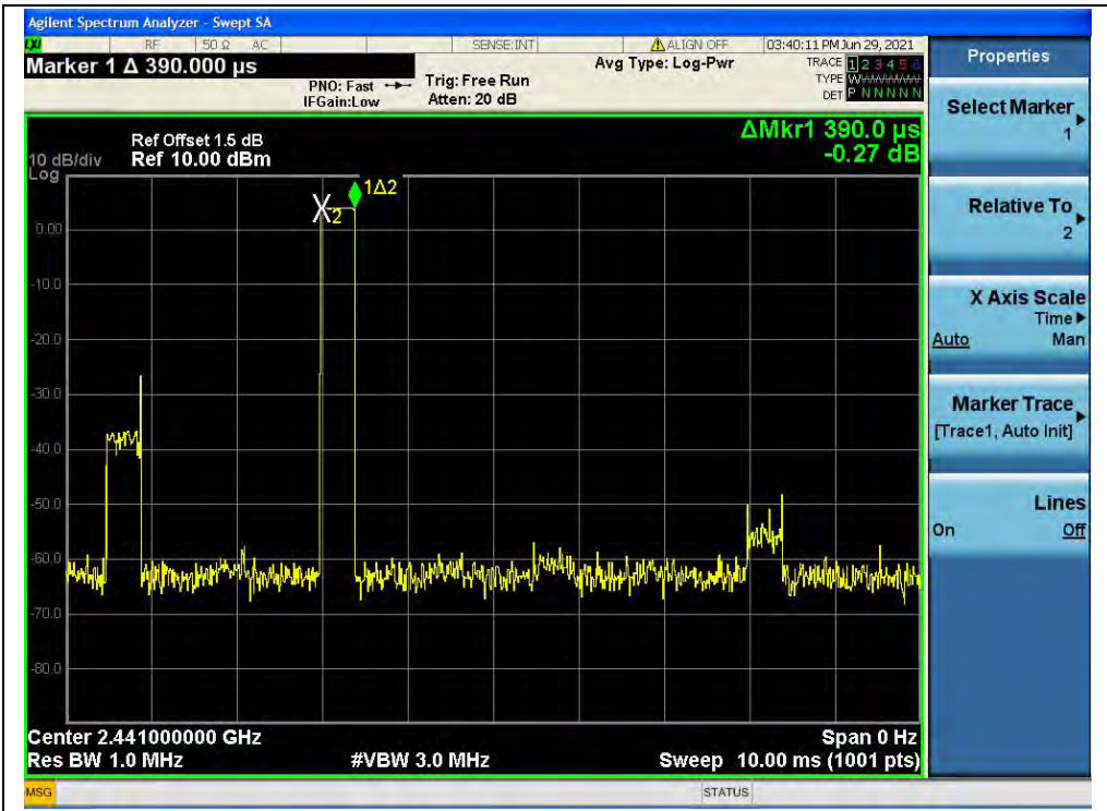
(DH1, GFSK)
