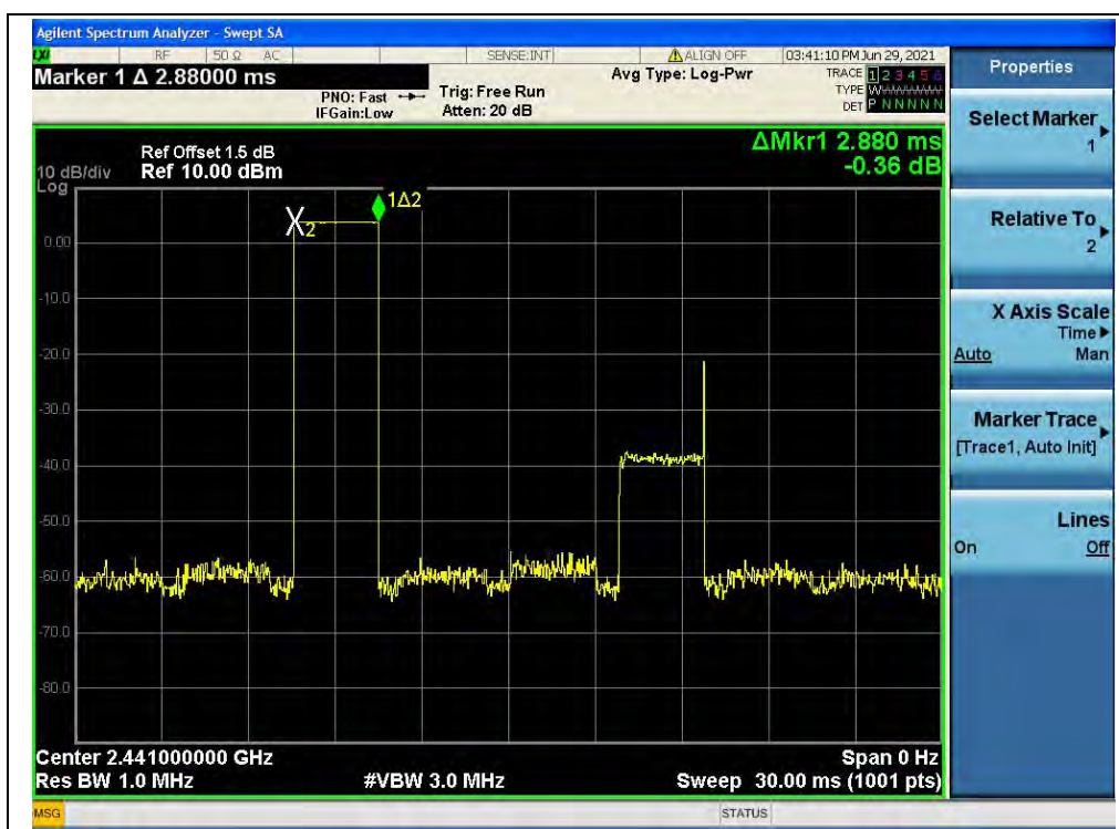
(DH5, GFSK)
