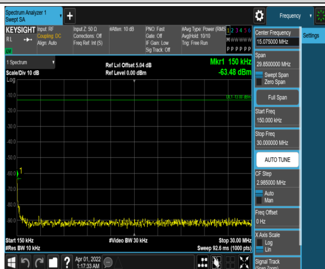
Band13-5MHz-QPSK-23255-1RB#0-Range2:0.15~30MHz
