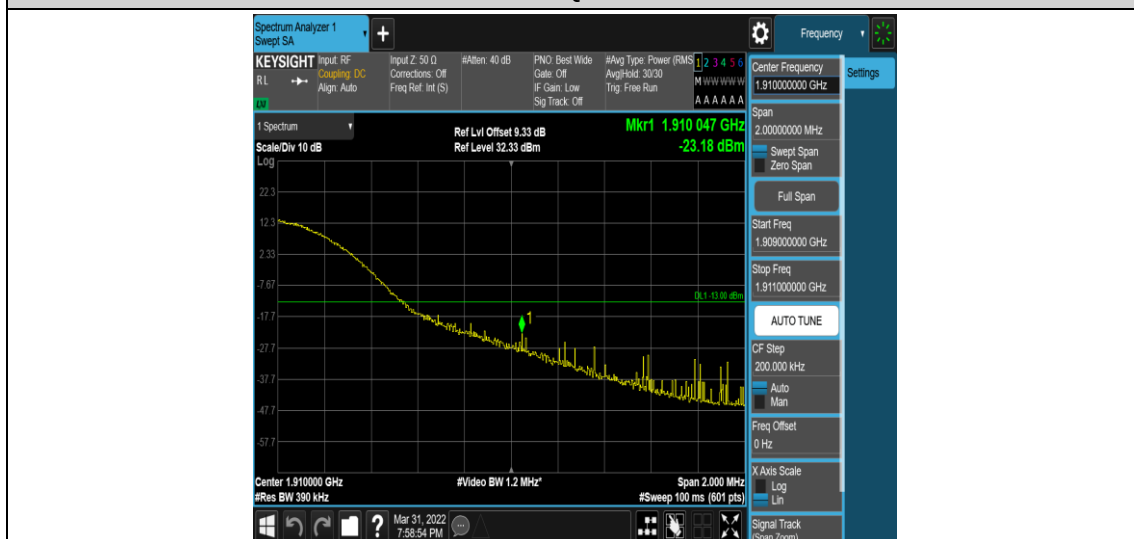
Band2-20MHz-16QAM-19100-1RB#99
