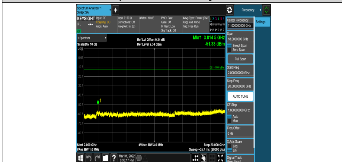
Band2-3MHz-QPSK-19185-1RB#0-Range5:2000~20000MHz
