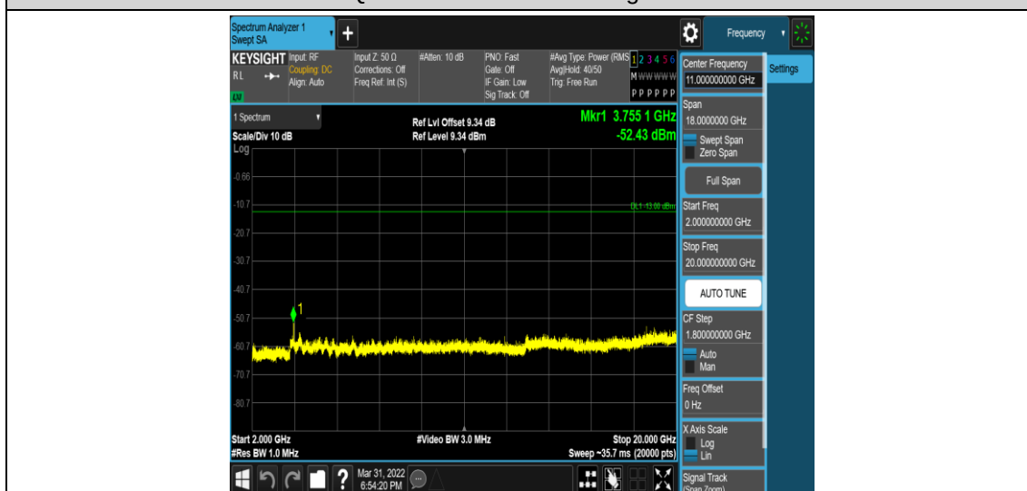
Band2-5MHz-QPSK-18900-1RB#0-Range5:2000~20000MHz
