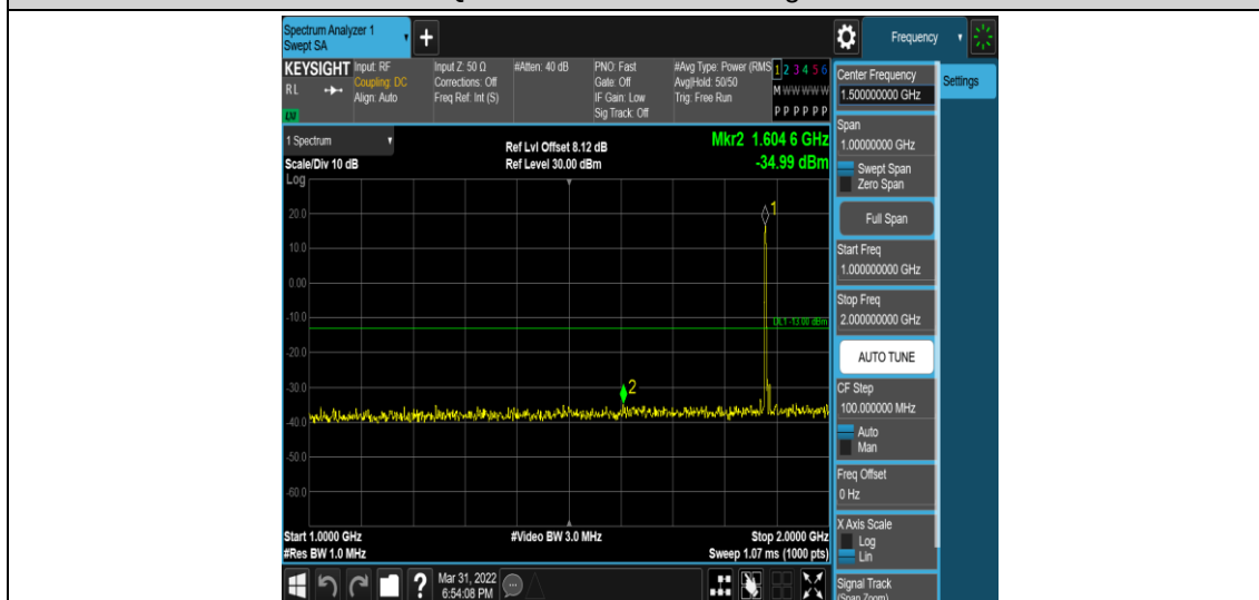
Band2-5MHz-QPSK-18900-1RB#0-Range4:1000~2000MHz
