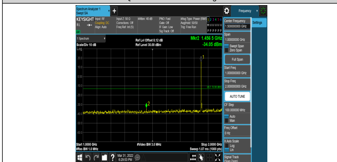
Band2-3MHz-16QAM-18615-1RB#0-Range4:1000~2000MHz
