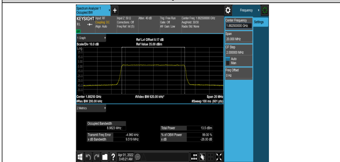
Band25-10MHz-16QAM-26365-50RB#0
