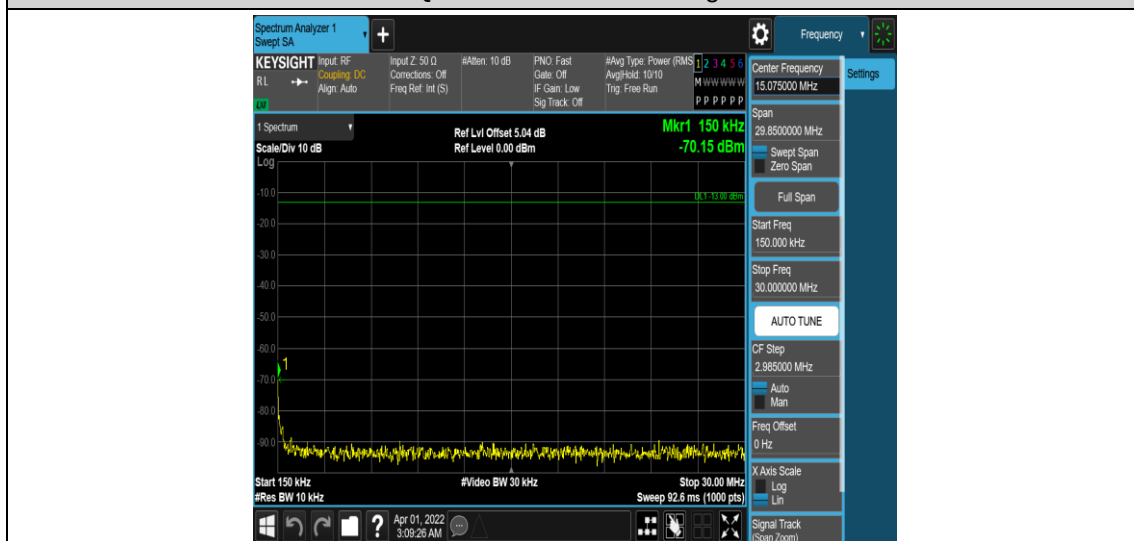
Band25-3MHz-16QAM-26365-1RB#0-Range2:0.15~30MHz
