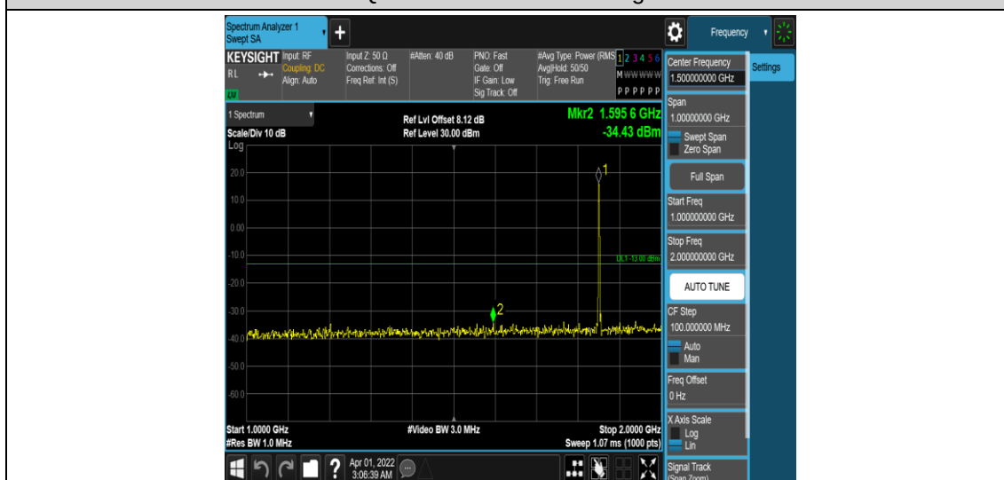
Band25-3MHz-QPSK-26055-1RB#0-Range4:1000~2000MHz
