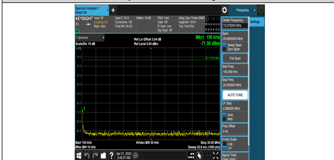
Band25-1.4MHz-16QAM-26365-1RB#0-Range2:0.15~30MHz
