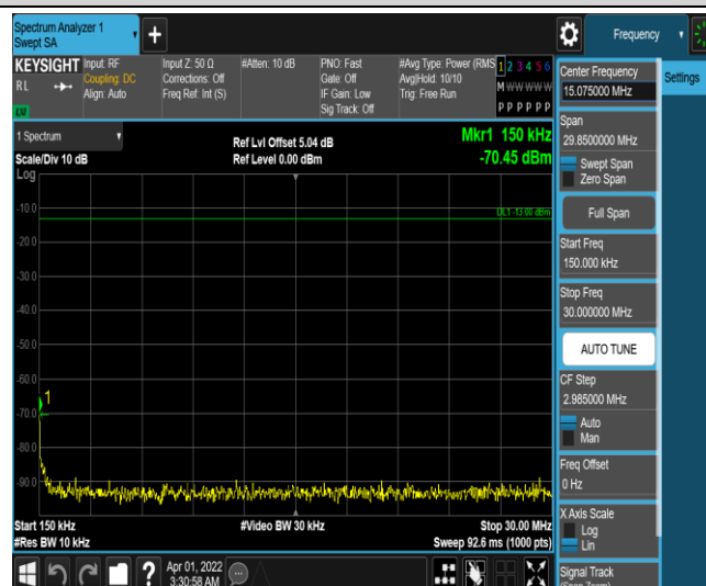
Band25-5MHz-QPSK-26365-1RB#0-Range2:0.15~30MHz
