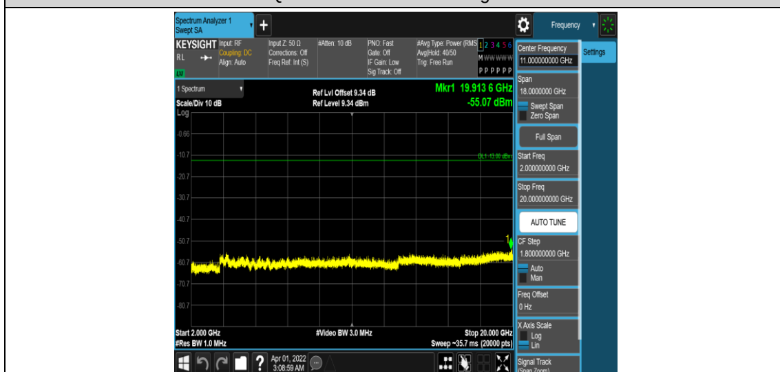
Band25-3MHz-QPSK-26365-1RB#0-Range5:2000~20000MHz
