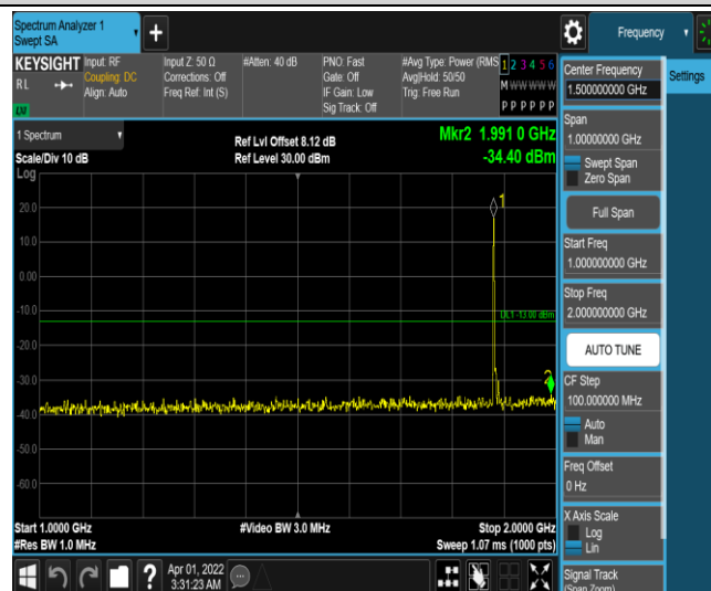
Band25-5MHz-QPSK-26365-1RB#0-Range4:1000~2000MHz
