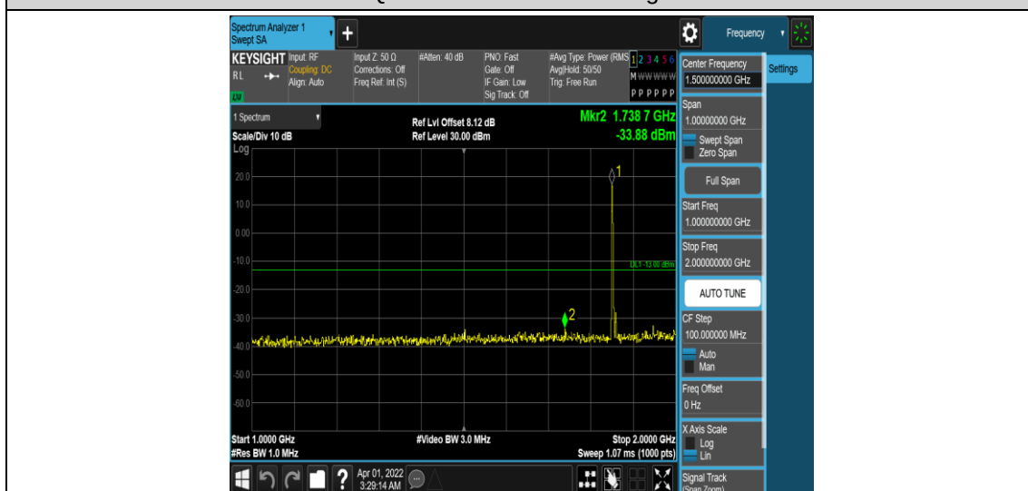
Band25-5MHz-QPSK-26065-1RB#0-Range4:1000~2000MHz
