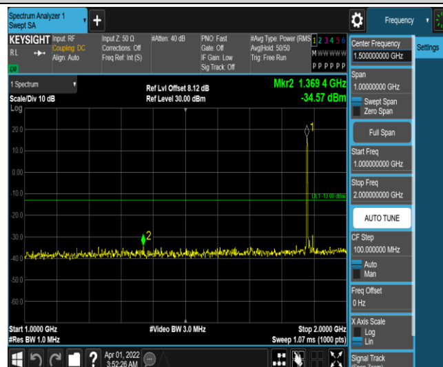
Band25-10MHz-QPSK-26365-1RB#0-Range4:1000~2000MHz
