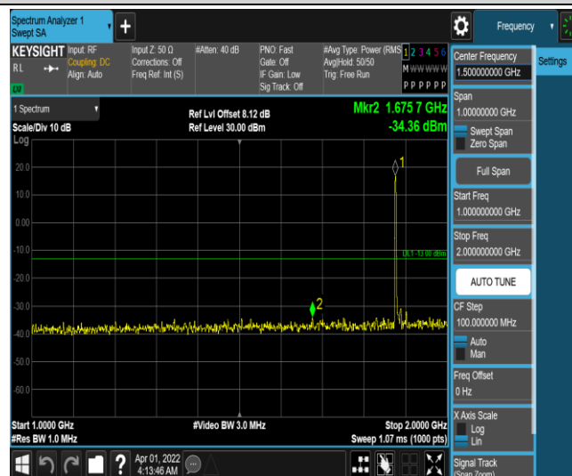
Band25-15MHz-QPSK-26365-1RB#0-Range4:1000~2000MHz
