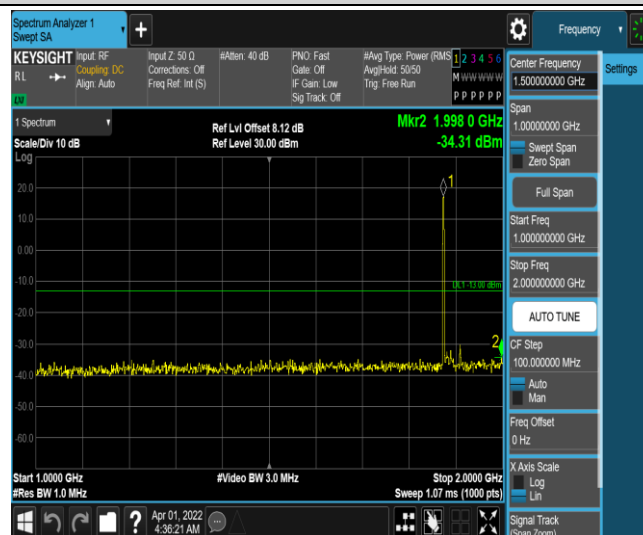
Band25-20MHz-16QAM-26365-1RB#0-Range4:1000~2000MHz
