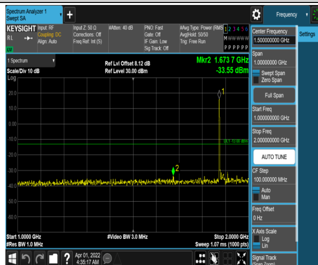
Band25-20MHz-QPSK-26365-1RB#0-Range4:1000~2000MHz
