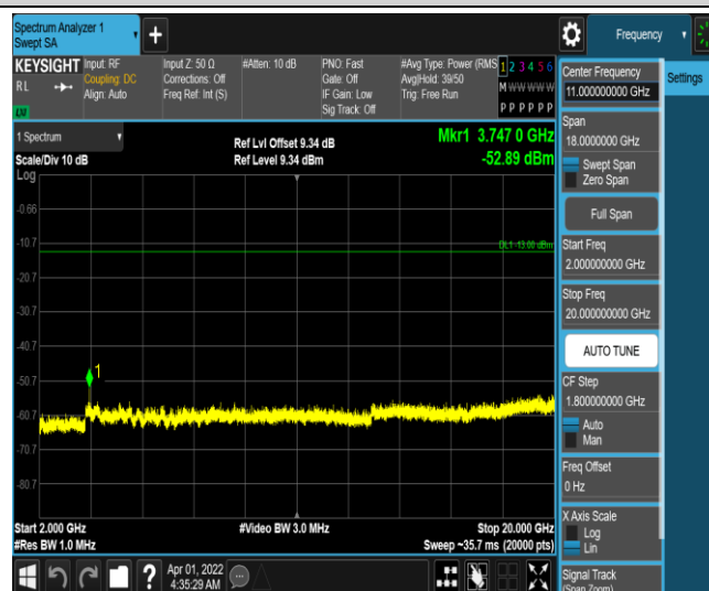
Band25-20MHz-QPSK-26365-1RB#0-Range5:2000~20000MHz
