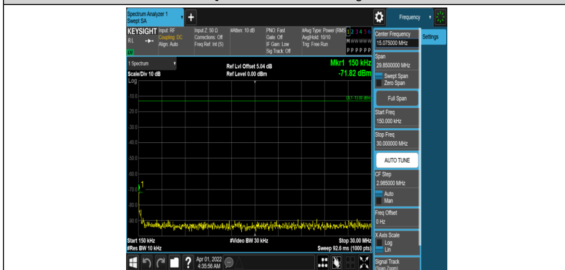
Band25-20MHz-16QAM-26365-1RB#0-Range2:0.15~30MHz
