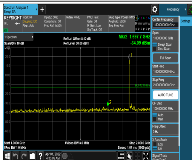
Band25-20MHz-QPSK-26140-1RB#0-Range4:1000~2000MHz
