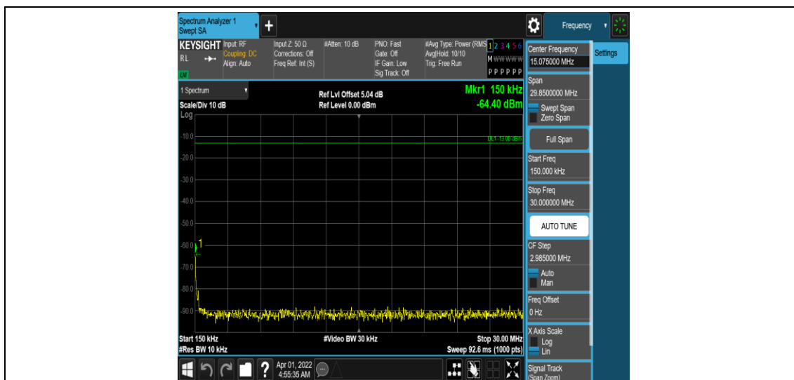
Band26-1.4MHz-QPSK-26740-1RB#0-Range2:0.15~30MHz
