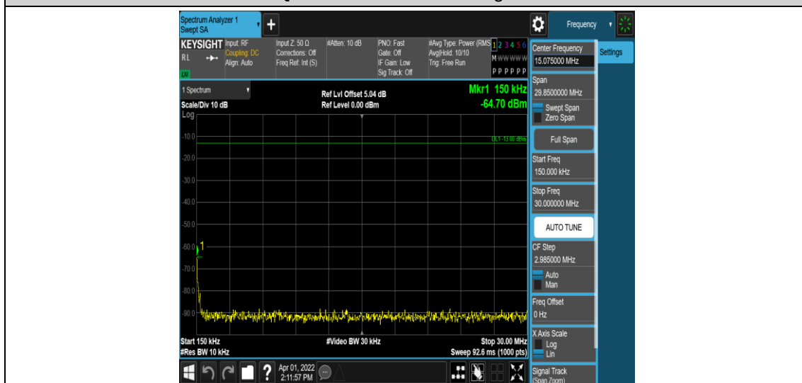
Band26-3MHz-QPSK-26805-1RB#0-Range2:0.15~30MHz
