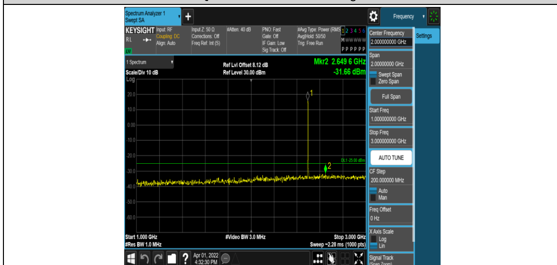
Band41-5MHz-QPSK-39675-1RB#0-Range4:1000~3000MHz
