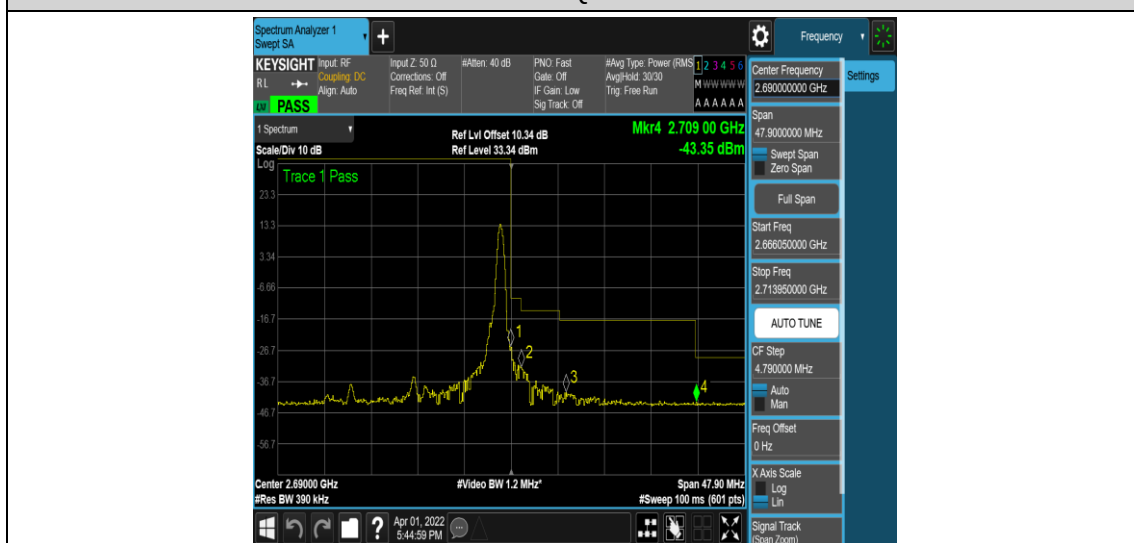
Band41-20MHz-16QAM-41490-1RB#99
