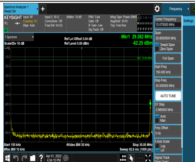
Band41-5MHz-QPSK-40620-1RB#0-Range2:0.15~30MHz
