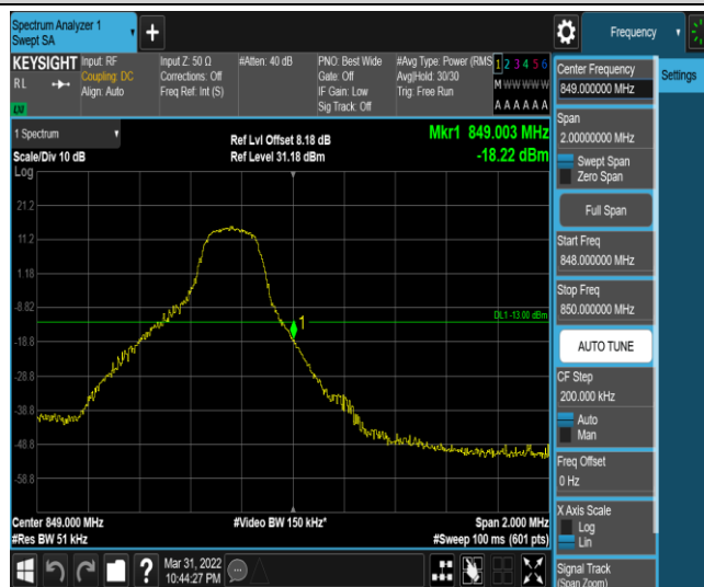
Band5-3MHz-QPSK-20635-1RB#14
