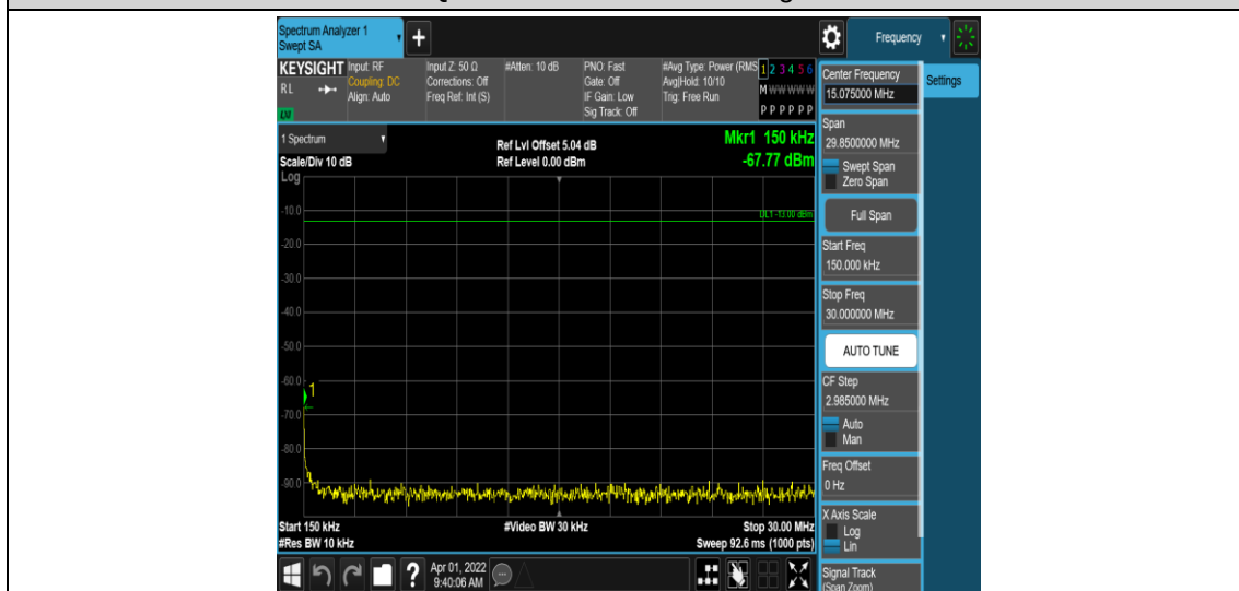
Band66-20MHz-QPSK-132572-1RB#0-Range2:0.15~30MHz
