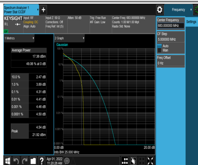
Band71-20MHz-QPSK-133322-1RB#0
