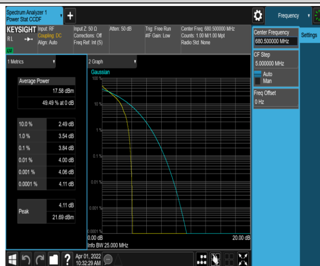
Band71-10MHz-QPSK-133297-1RB#0
