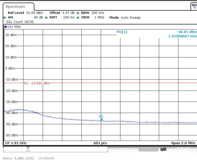
Band2-15MHz-16QAM-19125-1RB#74
