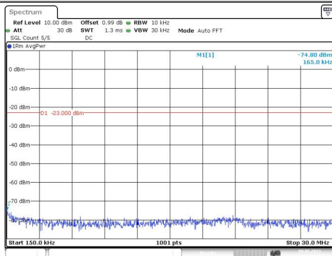
Band26-1.4MHz-QPSK-26697-1RB#0-Range2:0.15~30MHz
