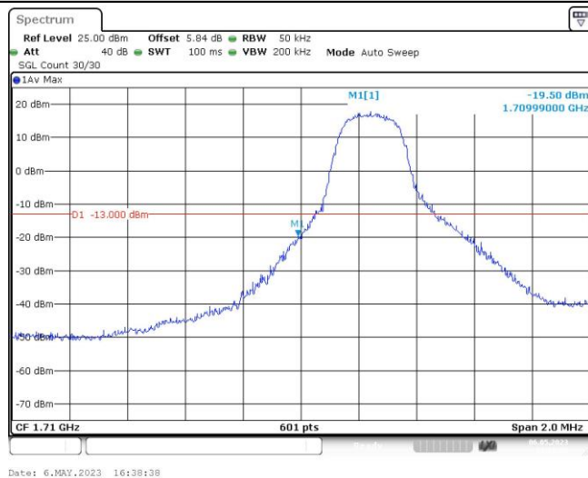
Band4-3MHz-QPSK-19965-1RB#14
