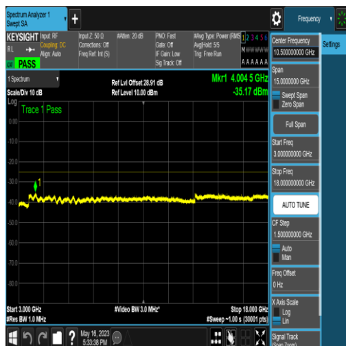
NTNV_N41_PC2_30_10_M_TID16_N/A_3000_18 000_#1
