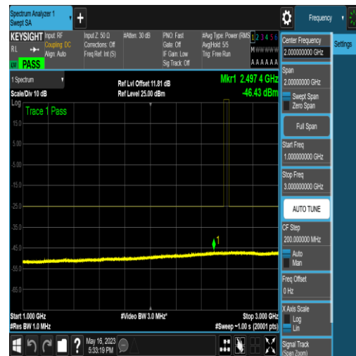
NTNV_N41_PC2_30_10_M_TID16_N/A_1000_30 00_#1
