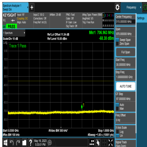
NTNV_N41_PC2_30_10_M_TID16_N/A_30_1000 _#1
