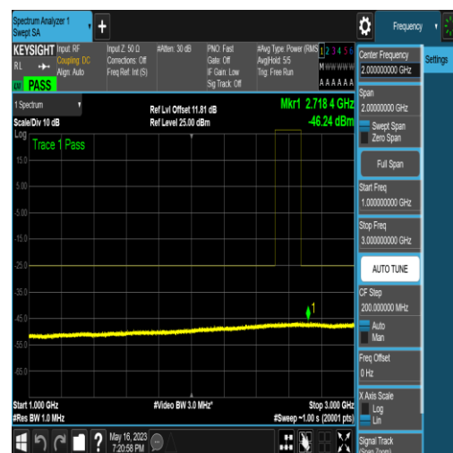
NTNV_N41_PC2_30_50_M_TID17_N/A_1000_30 00_#1
