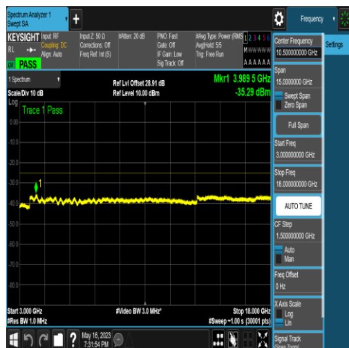
NTNV_N41_PC2_30_60_L_TID6_N/A_3000_180 00_#1
