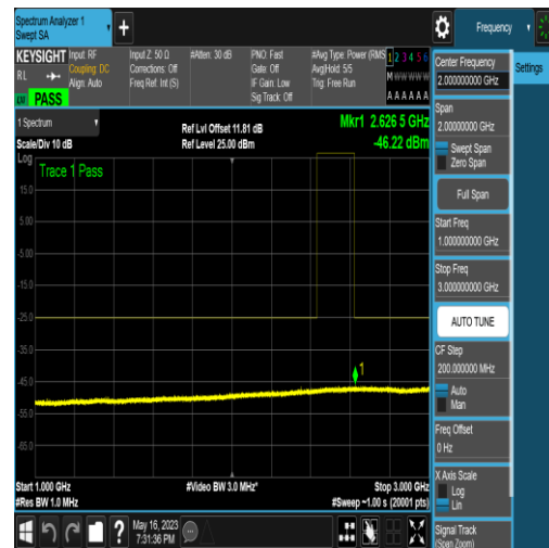
NTNV_N41_PC2_30_60_L_TID6_N/A_1000_300 0_#1
