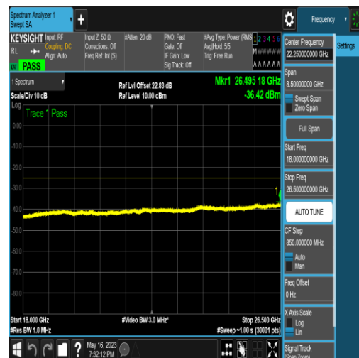
NTNV_N41_PC2_30_60_L_TID6_N/A_18000_26 500_#1
