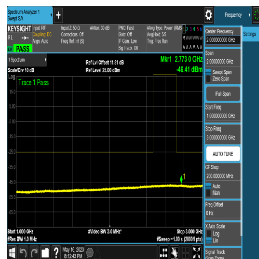
NTNV_N41_PC2_30_80_M_TID16_N/A_1000_30 00_#1
