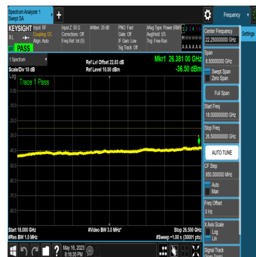
NTNV_N41_PC2_30_80_H_TID6_N/A_18000_26 500_#1
