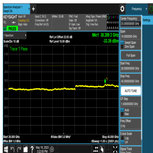
NTNV_N77-3450-3550_PC2_30_50_L_TID6_N/A _26000_40000_#1
