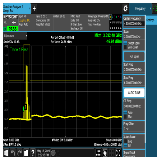
NTNV_N77-3450-3550_PC2_30_50_L_TID6_N/A _3000_6000_#1
