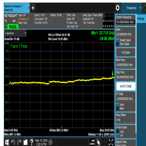
NTNV_N77-3450-3550_PC2_30_50_L_TID6_N/A _6000_26000_#1
