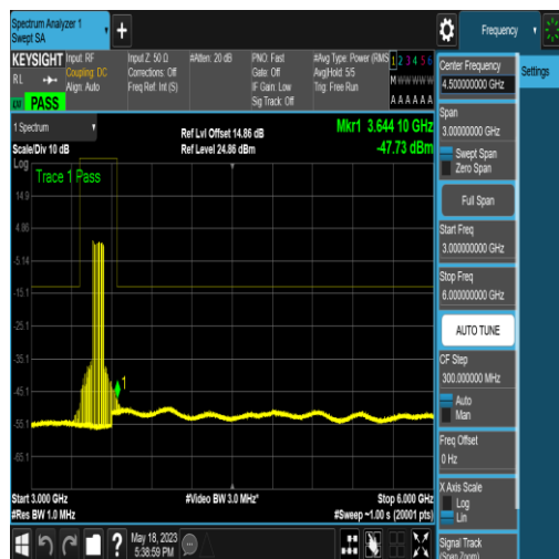
NTNV_N77-3450-3550_PC2_30_90_M_TID6_N/A _3000_6000_#1
