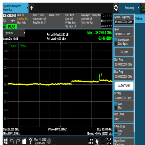
NTNV_N77-3450-3550_PC2_30_20_L_TID6_N/A _26000_40000_#1
